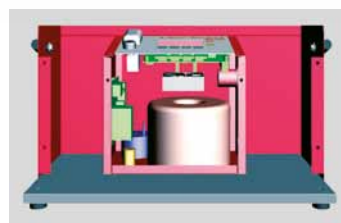
Systém aktívneho chladenia (AC)! Zvýšenie výkonu o 20% pri sériových zvaroch. Neexistuje žiadna chyba zvärania v dôsledku prehriatia
