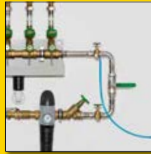
Nyomáspróba sűrített levegővel (SL/SLW)
