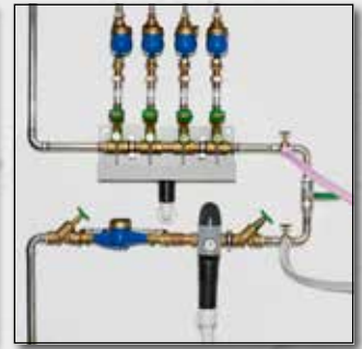
Ivóvízrendszerek öblítése (S/SL/SLW)
